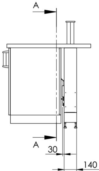
Ausschnitt für Steuerung mittig Hubhaube in Küchenschrank-Rückwand
